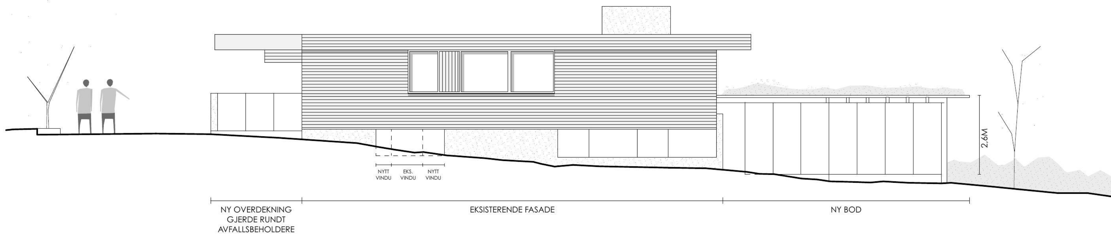
FASADE NORDVEST
